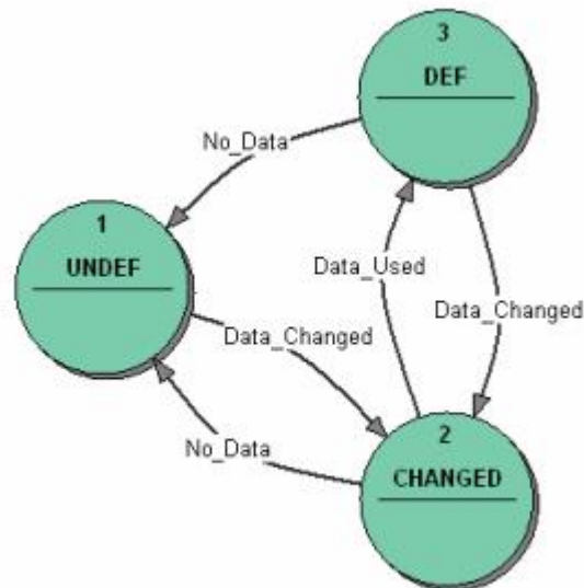
Figure 15: DAT VFSM
