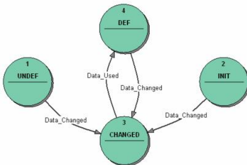
Figure 20: PAR VFSM
